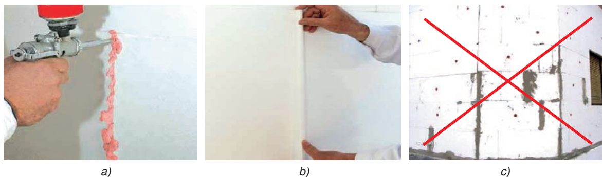
Slika 2-30 Ispunjavanje fuga između ploča toplinske izolacije: a) PUR pjenom, b) istim izolacijskim materijalom, c) primjer lošeg izvođenja - ljepilo u fugama [10]
