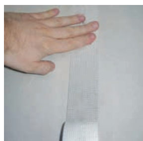
Slika 4-48 Postava bandažne trake na spojeve ploča [190]
