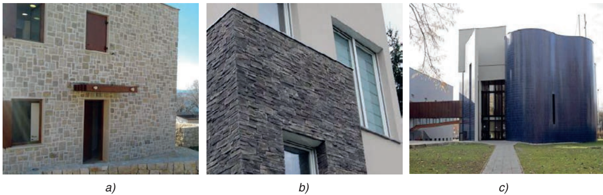
Slika 2-78 Obloga ETICS sustava s: a) prirodnim kamenom; b) umjetnim kamenom; c) keramikom [19], [118]
