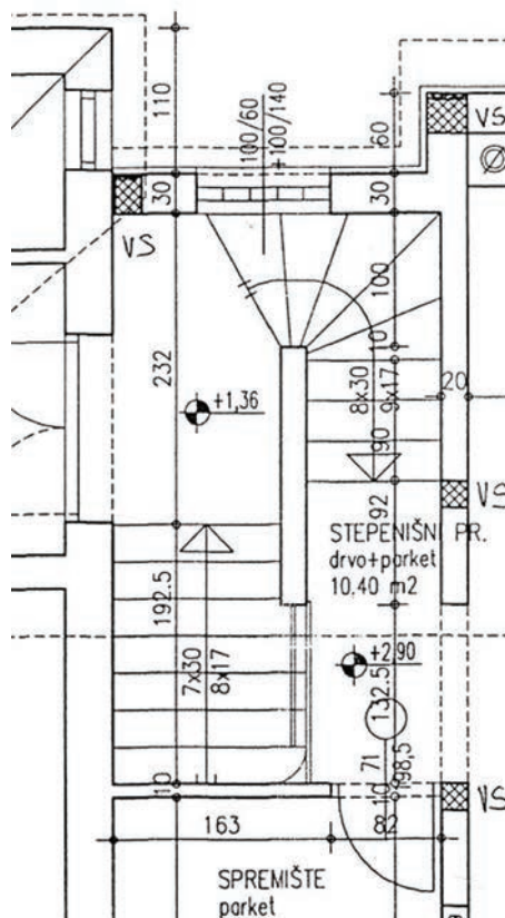
Slika 4-6 Primjer tlocrta stubišta M 1:50
