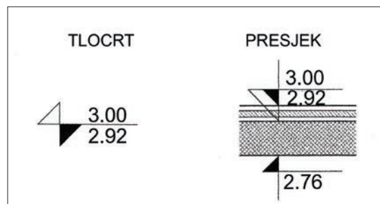
Slika 4-22 Oznake visinskih kota
