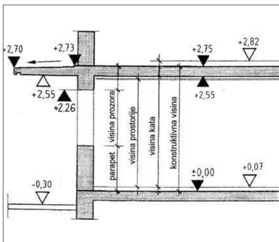
Slika 4-25 Dimenzije koje se kotiraju u presjeku
