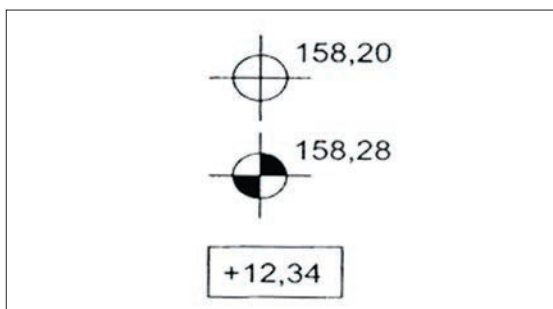
Slika 4-23 Oznake visinskih kota u tlocrtu
