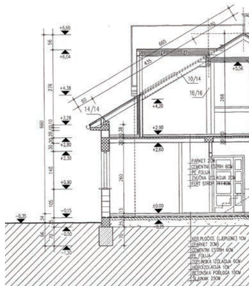
Slika 4-10 Presjek M 1:50
