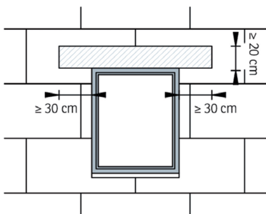
Slika 3-19 Protupožarna barijera u visini natprozornika [31]
