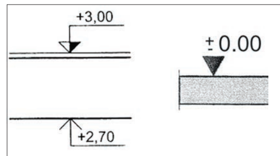
Slika 4-24 Oznake visinskih kota u presjeku
