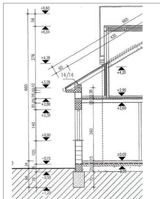
Slika 4-26 Kotiranje u presjeku
