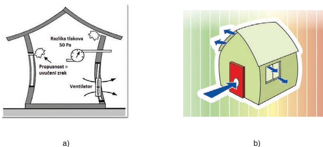
Slika 5-28 Shematski prikaz postupka mjerenja zrakopropusnosti zgrade: a) ispuhivanje (podtlak); b) napuhavanje (nadtlak) [171], [172]
