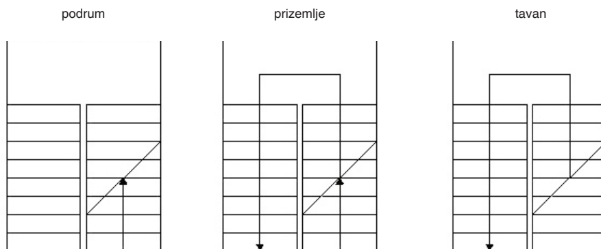
Slika 4-5 Prikaz stubišta u tlocrtu
