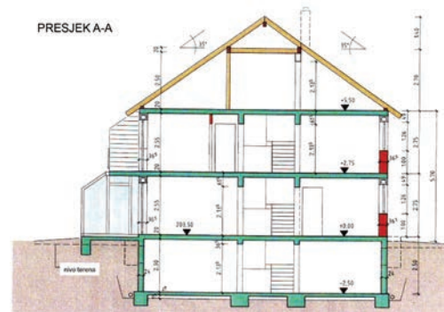
Slika 4-9 Presjek M 1:100
